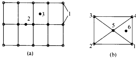
图 2 矩形或方形布孔法
